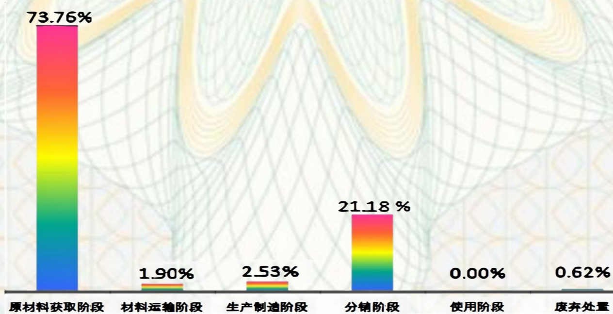
产品各生命周期阶段对碳足迹的贡献比例
